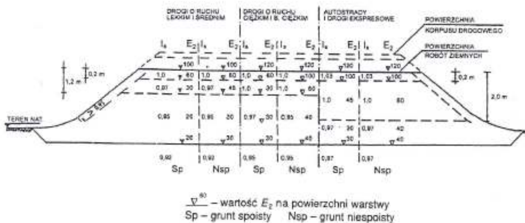
Rysunek 3 – Wartości wymagane w nasypach: Wskaźnika zagęszczenia I_2 i wtórnego modułu odkształcenia E_2 , megapaskali
