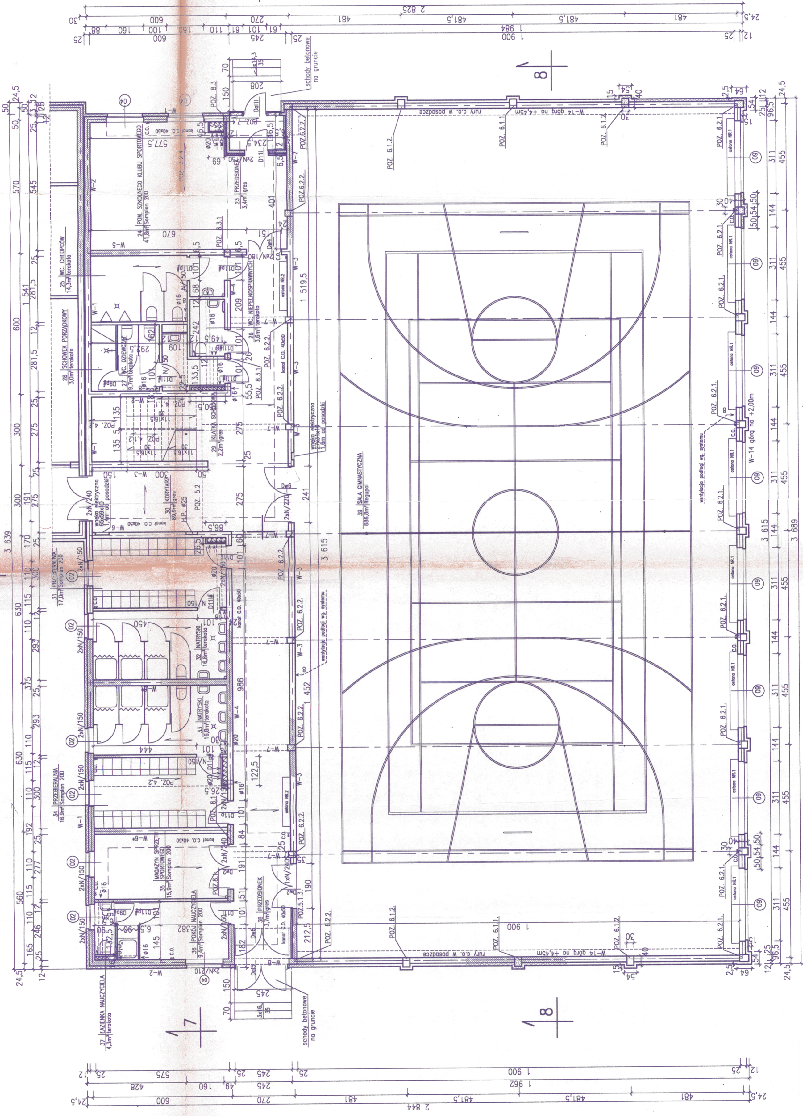
RZUT PARTERU 1:100
